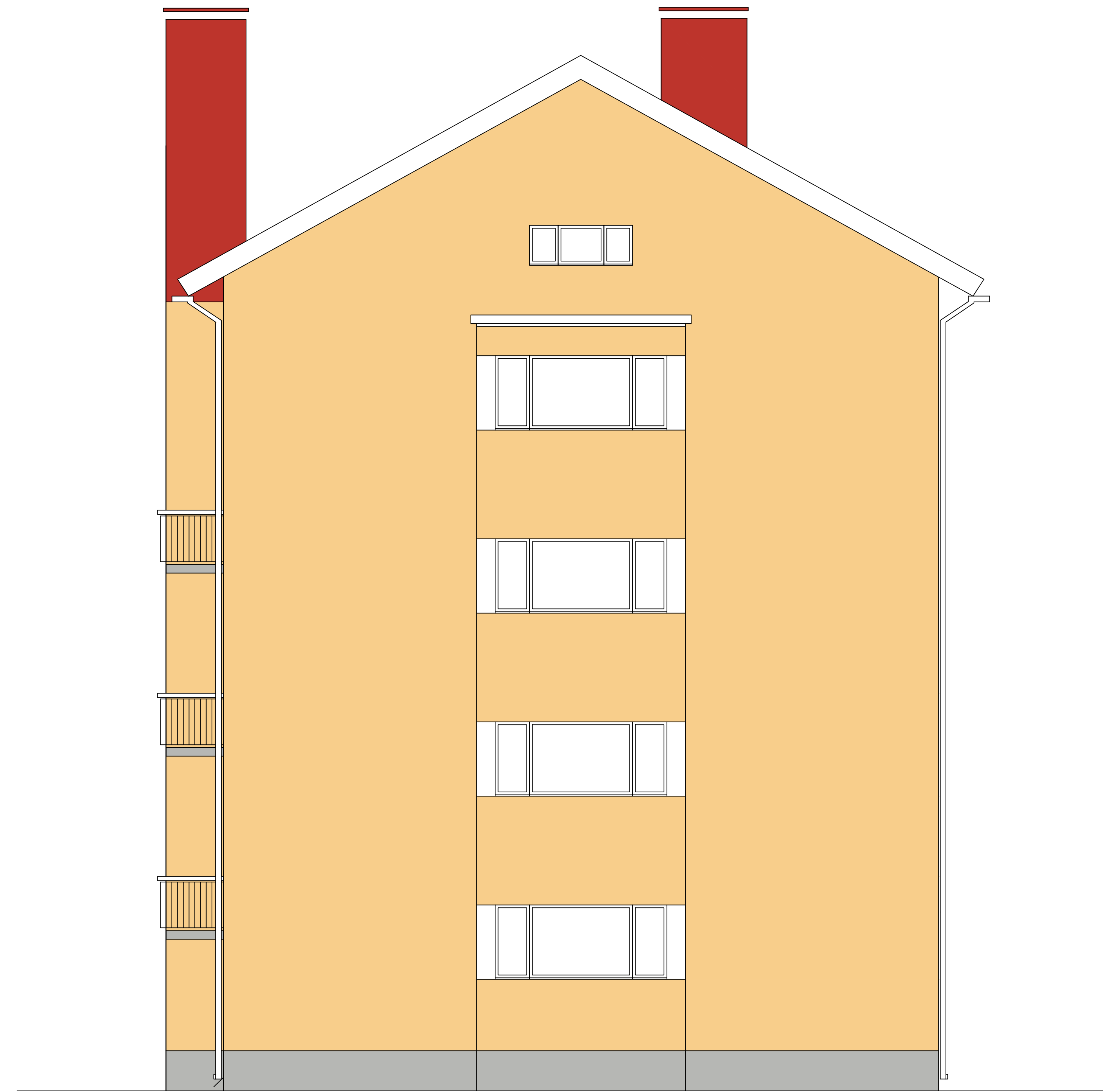
JULKISIVU KOILLISEEN mk 1:50
