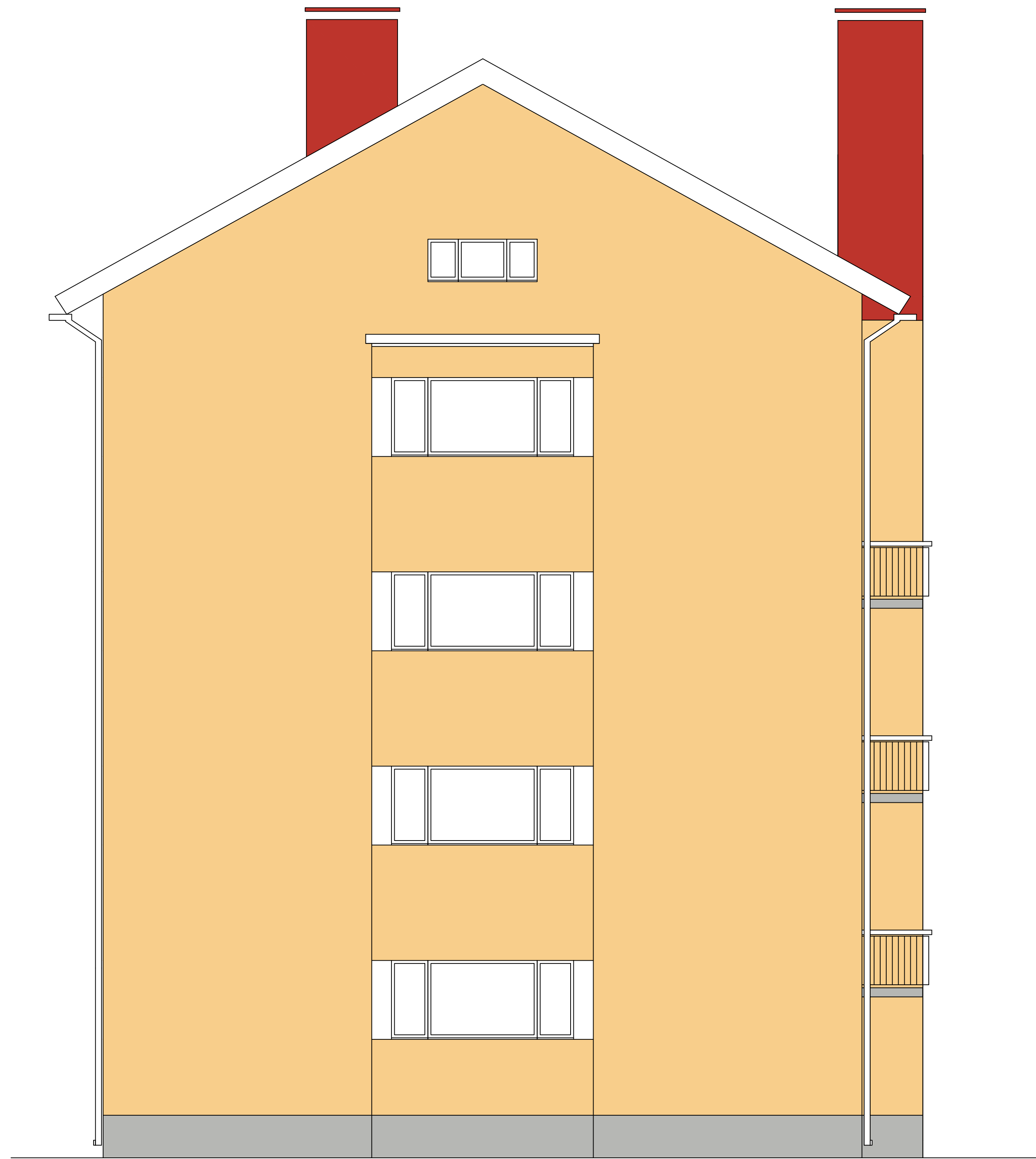
JULKISIVU LOUNAASEEN mk 1:50
