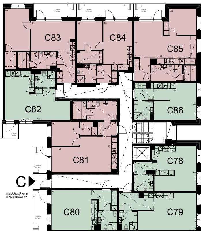
3. KERROS
