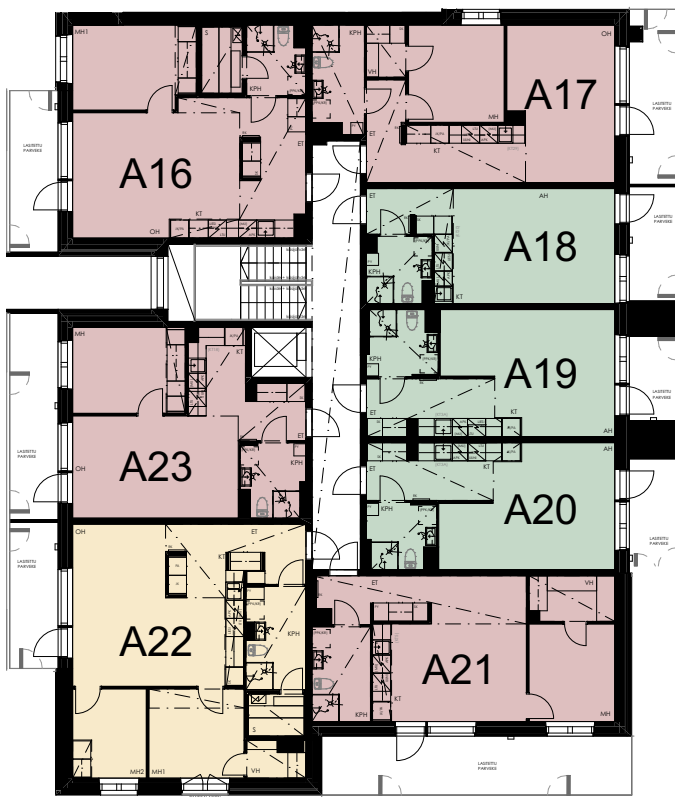
5. KERROS
