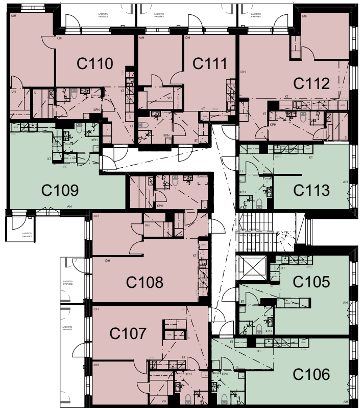
6. KERROS
