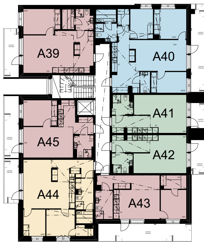
8. KERROS
