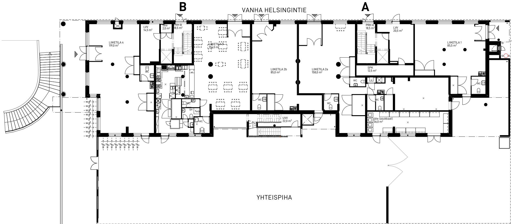
VHT 20 Kerrosphoja, 1. kerros 1:250
