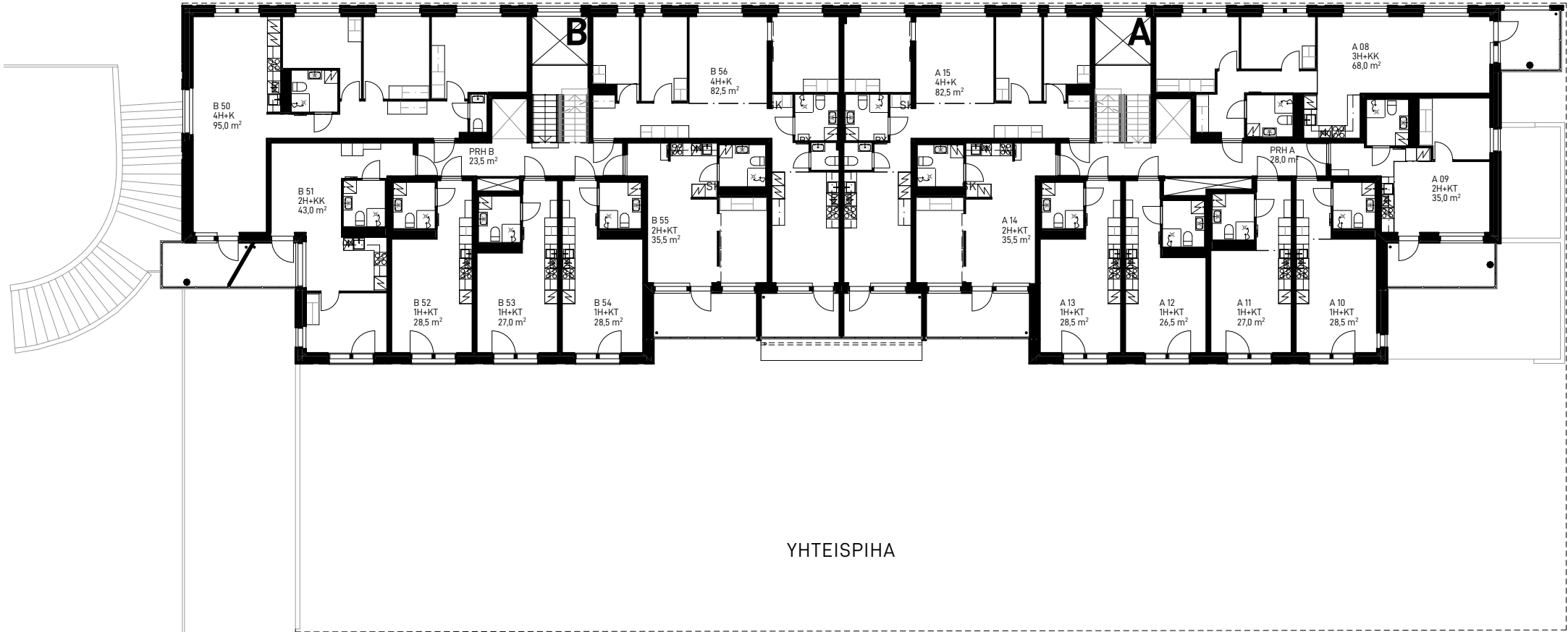
VHT 20 Kerrosphoja, 3. kerros 1:250
