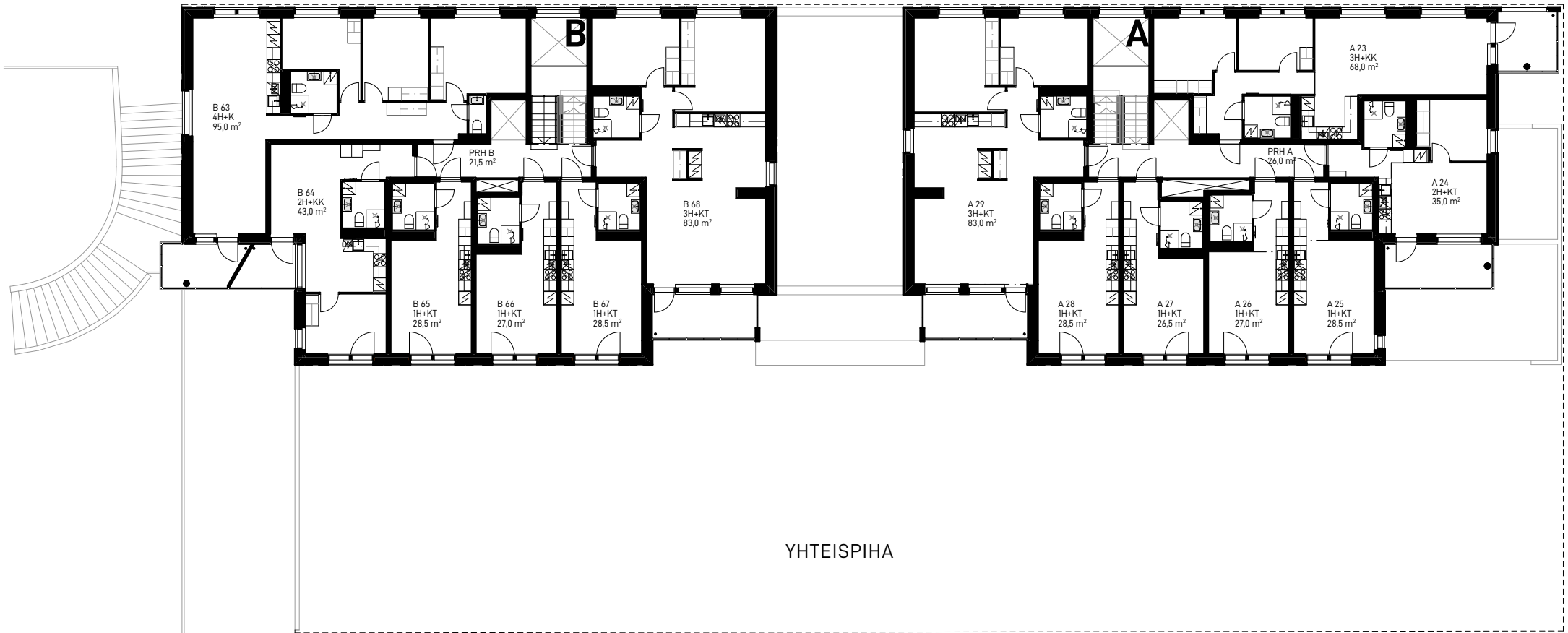
VHT 20 Kerrosphja, 5. kerros 1:250
