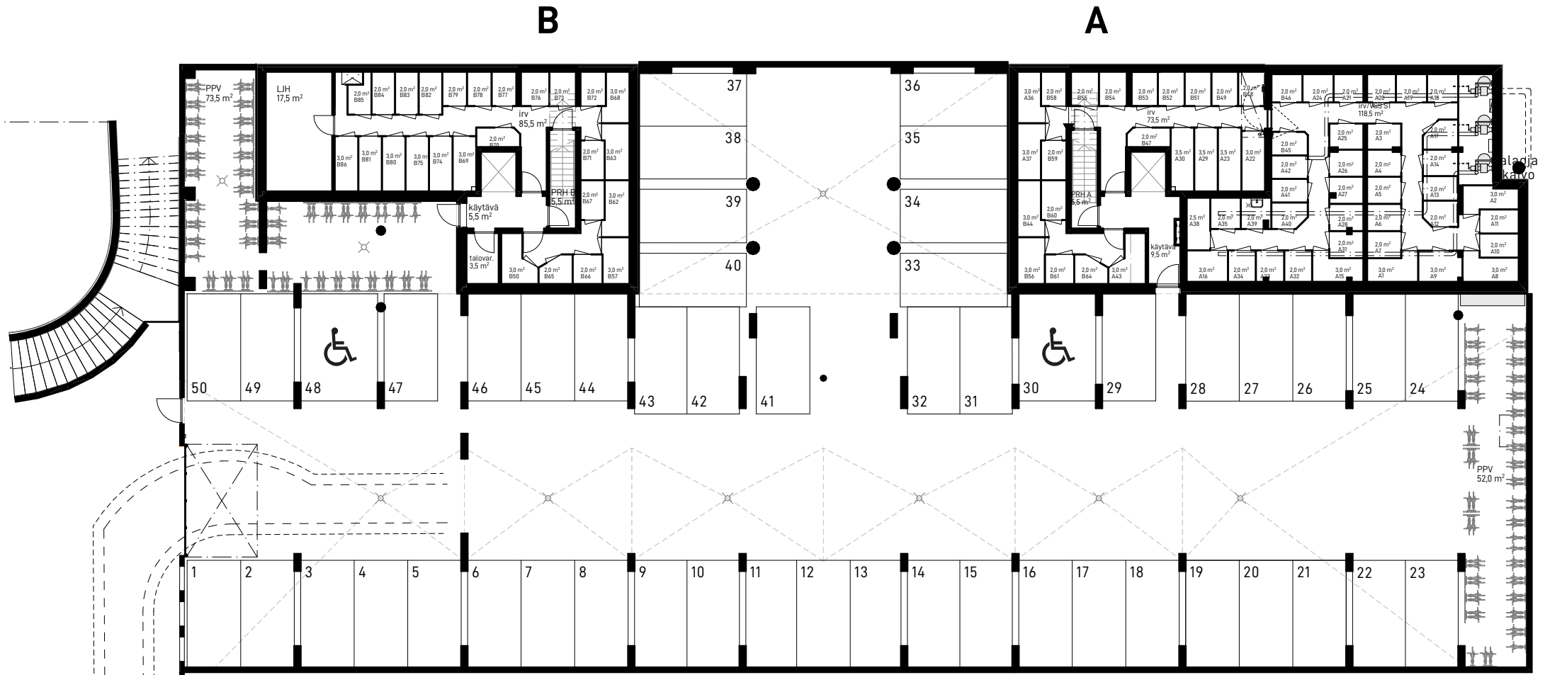
VHT 20 Kerrosphoja, kellarit 1:250
