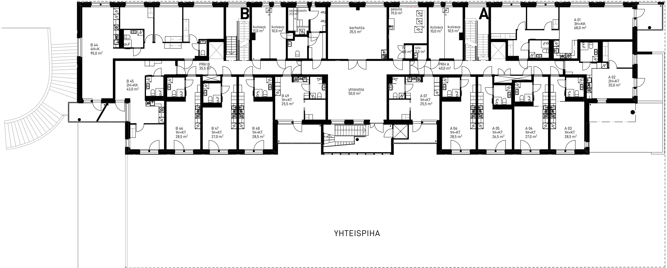
VHT 20 Kerrosphoja, 2. kerros 1:250
