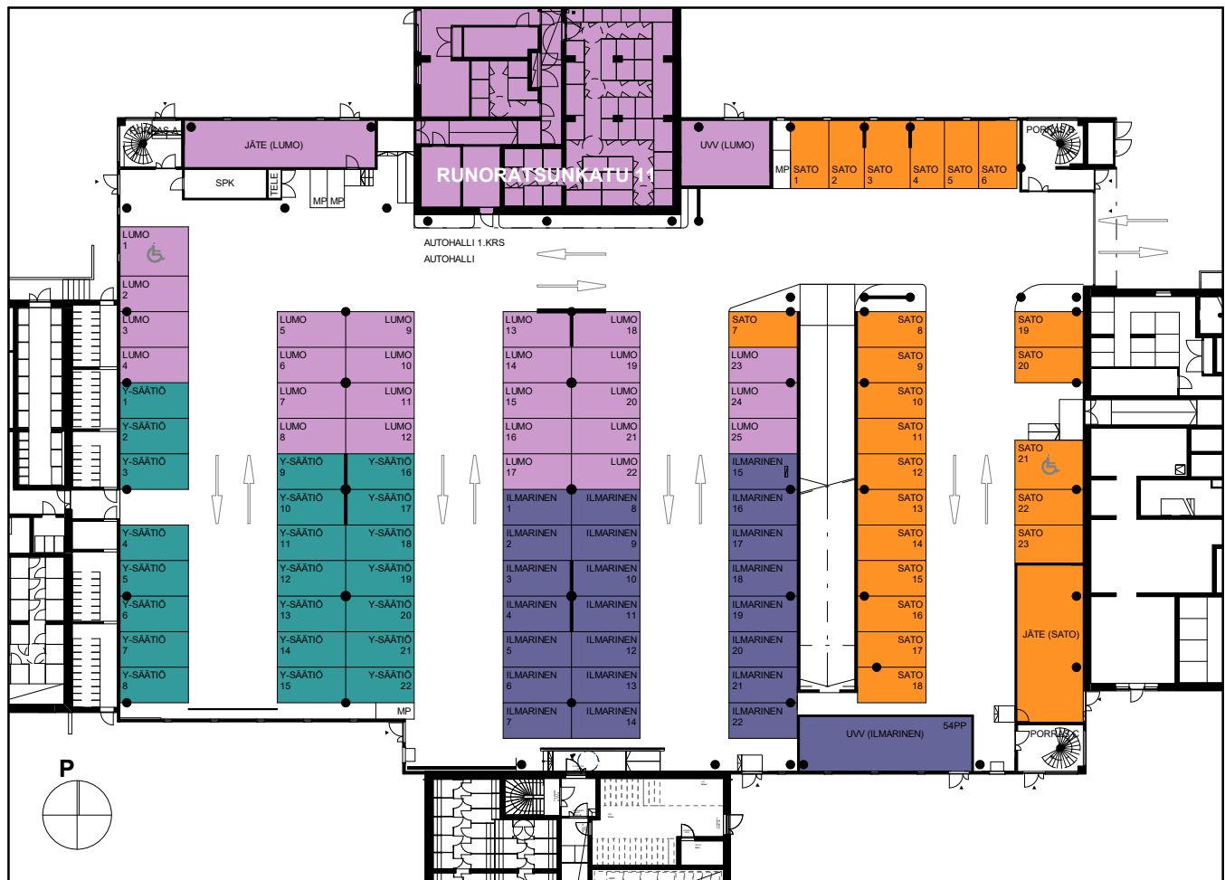
POHJA, 1-KERROS
